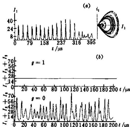
图2 根据方程(1)和(2), 取 \beta = 0.26 , 数值计算
