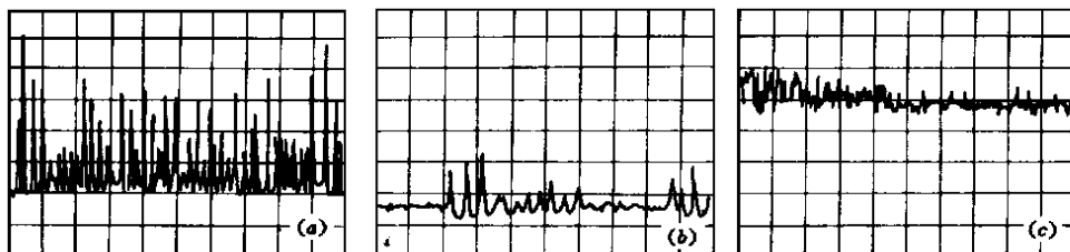
图3 实验记录的激光波形
