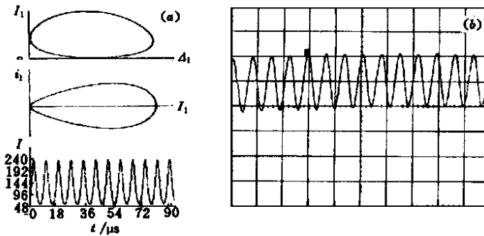
图 4 加入 Nd:YAG 色心调制晶体后, 混沌被消除
