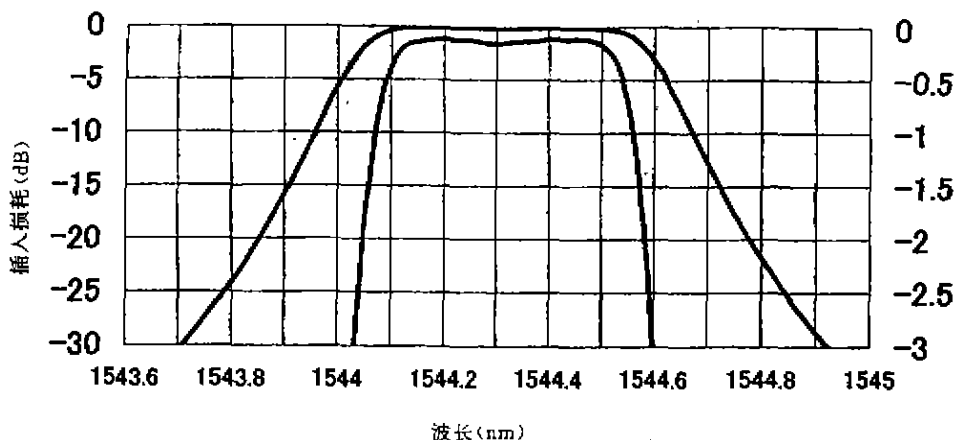
图 5 4 腔结构 100GHz DWDM 滤光片的实测曲线
