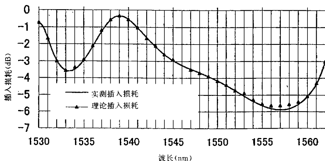
图 6 增益平坦滤光片曲线
