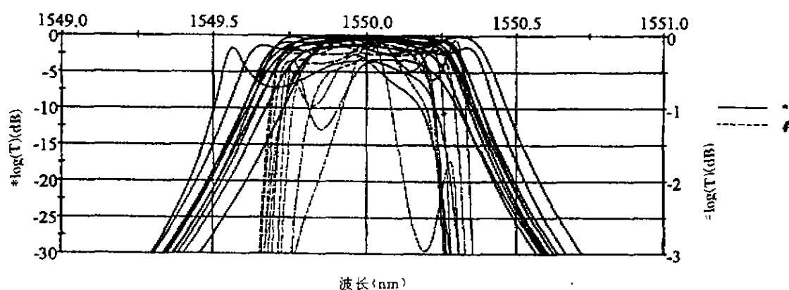
图2 膜厚误差的标准方差为 1 \times 10^{-4} 时的结果
