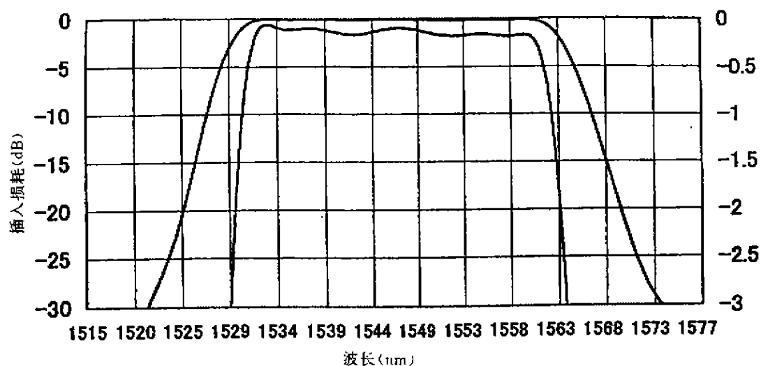
图 7 CWDM 的滤光片曲线
