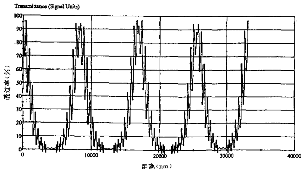
图 4 直接监控信号模拟
