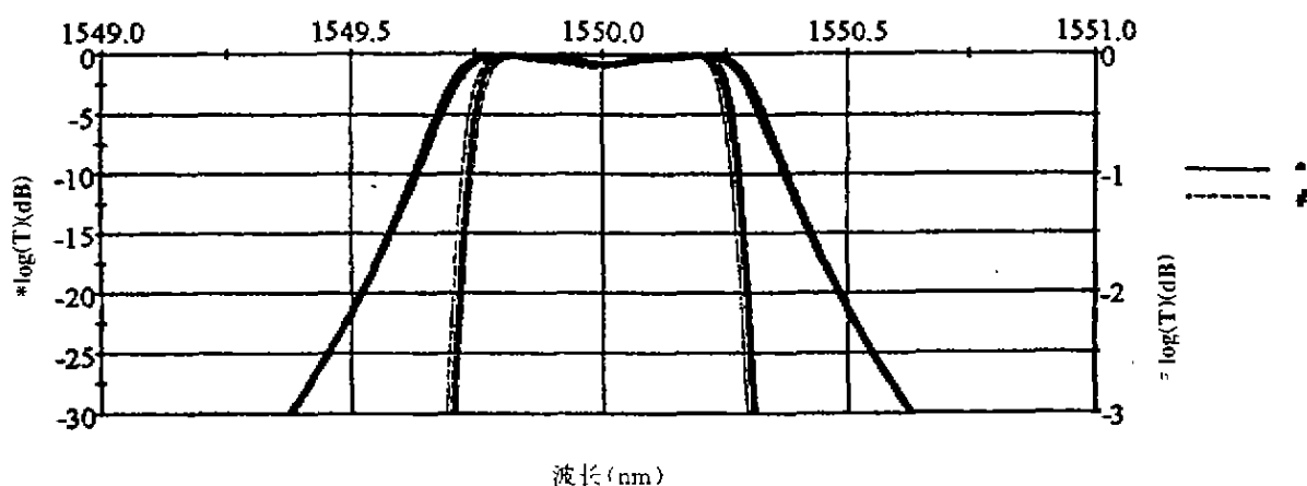
图3 膜厚误差的标准方差为 1 \times 10^{-5} 时的结果
