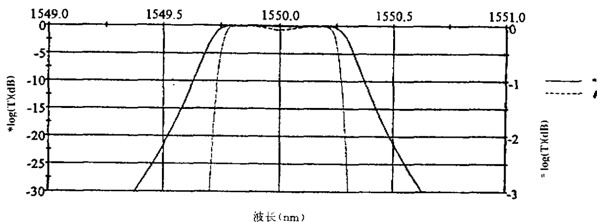
图1 4层结构100GHzDWDM滤光片的设计曲线
