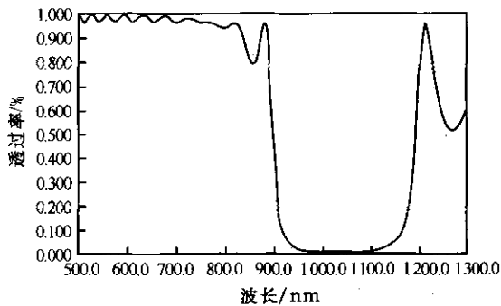
图1 短波通滤光片波长-透过率曲线
