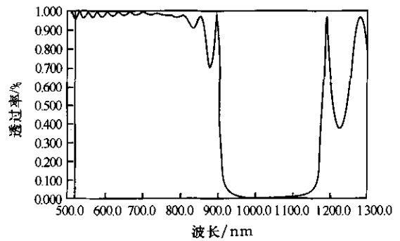
图2 改进后的短波通滤光片透过率曲线
