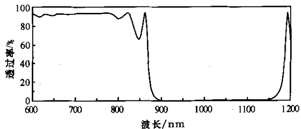
图3 短波通滤光片测试结果
