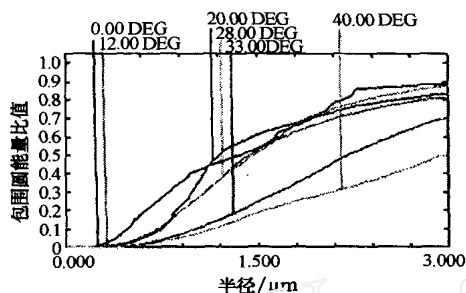
图2 能量集中度曲线
