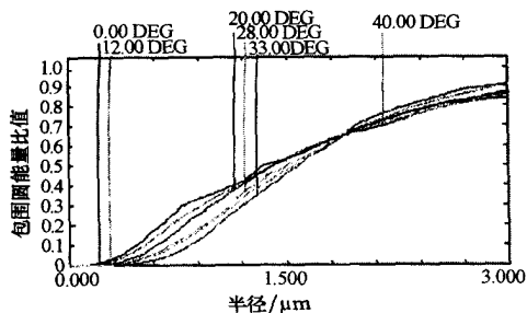
图4 采用非球面镜头的能量集中度曲线
