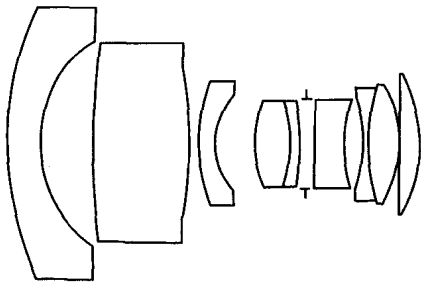
图1 镜头的初始结构示意图
