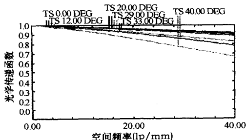
图3 光学传递函数
