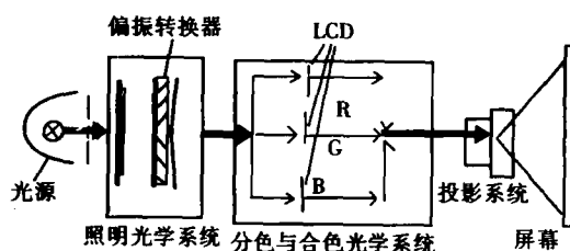
图1 液晶投影光学系统示意图
