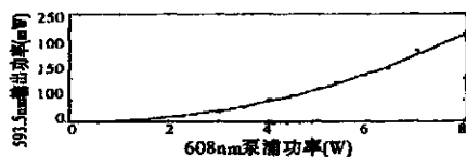
图 2 593.5nm 和频激光输出功率随入射泵浦功率变化关系
