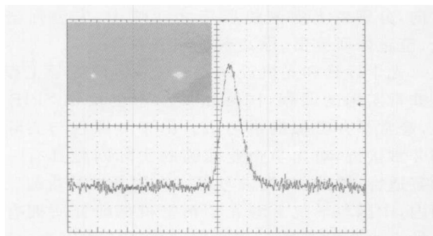
图3 深紫外213 nm激光脉冲波形 (插图为120 cm处拍摄的213 nm(左), 266 nm(右)激光输出模式)
