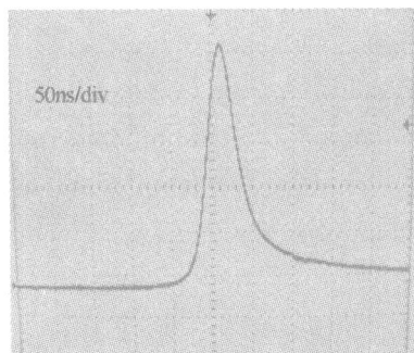
图 7 典型的脉冲波形 Fig. 7 The typical profile of SHG pulse
