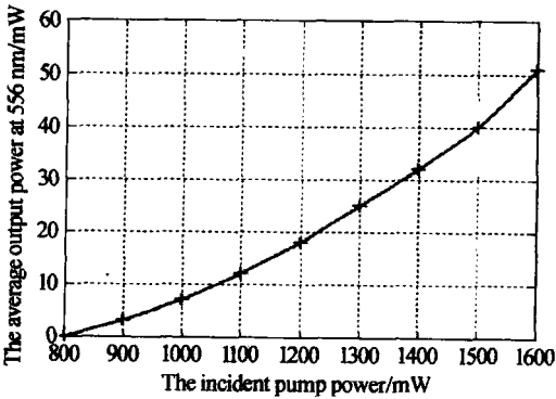
图 4 黄光的输出功率随输入功率的变化曲线 Fig. 4 The output power at the 556nm versus the pump power
