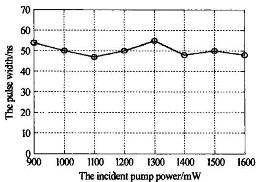
图 5 脉冲宽度随泵浦功率的变化曲线 Fig. 5 The pulse width versus the pump power
