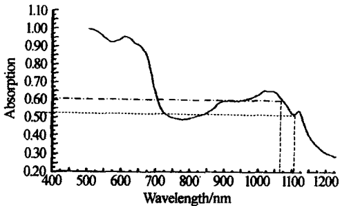
图 3 Cr :YAG 的吸收光谱 Fig. 3 The absorption spectrum of Cr :YAG
