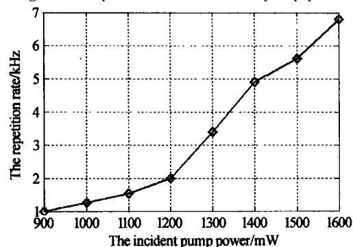
图 6 脉冲的重复频率随泵浦功率的变化 Fig. 6 The repetition rate versus the pump power
