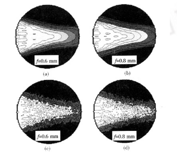
图 4 单侧面 5 个 bar 泵浦模拟结果
