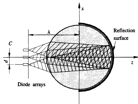
图 1 二极管阵列单侧面泵浦示意图
