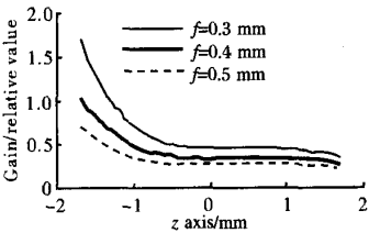
图 5 不同泵浦距离时阵列(5 个 bar)单侧面泵浦 z 轴泵浦光强度分布曲线图( r=1.75\text{ mm} , \alpha=0.4\text{ mm}^{-1} , \omega_0=1\text{ }\mu\text{m} )
