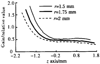
图 7 不同晶体半径时阵列(5 个 bar)单侧面泵浦 z 轴泵浦光强度分布曲线图( f=0.3\text{ mm} , \alpha=0.4\text{ mm}^{-1} , \omega_0=1\text{ }\mu\text{m} )
