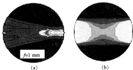
图 11 泵浦光分布示意图
