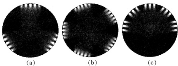
图 9 多侧面泵浦晶体的泵浦光强分布示意图( f=0.5\text{ mm} , r=2.5\text{ mm} , \alpha=0.4\text{ mm}^{-1} , \omega_0=1\text{ }\mu\text{m} )
