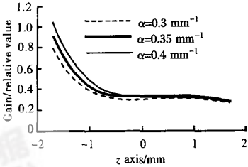
图 6 不同吸收系数条件下阵列(5 个 bar)单侧面泵浦 z 轴泵浦光强度分布曲线图( r=1.75\text{ mm} , f=0.4\text{ mm} , \omega_0=1\text{ }\mu\text{m} )
