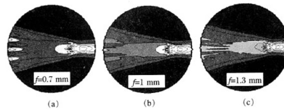
图 3 单侧面 5 个 bar 泵浦(一侧镀反射膜)
