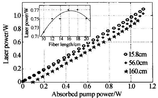
图 4 Tm2Ho 共掺石英光纤输出激光功率随泵浦功率的变化
