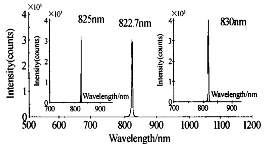
图 5 Tm2Ho 共掺石英光纤的输出光谱
