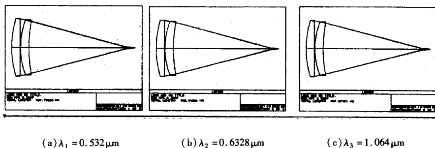
图 1 适用于不同波长的扩束器系统
