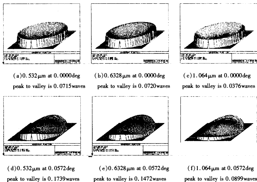
图 2 三种波长不同视场的波前图
