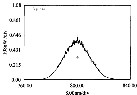
图 4 钛宝石激光器输出光谱图
