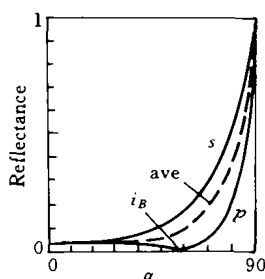
图 1 光波在玻璃表面的反射率
