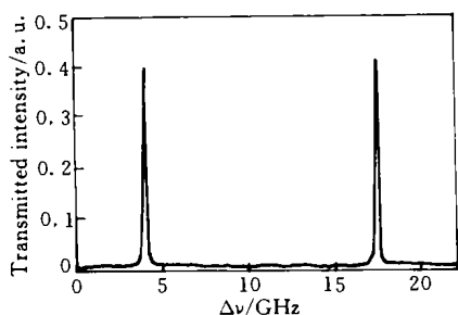
图 4 连续单频绿光激光器纵模扫描
