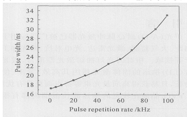
图 3 532 nm 激光脉冲宽度随重复频率的变化
