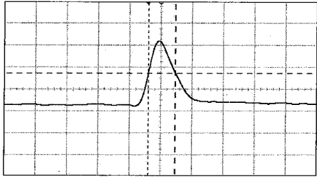
图 4 532 nm 调 Q 脉冲波形
