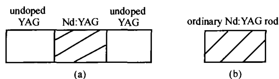
图 4 YAG 棒结构
