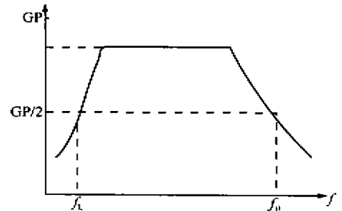
图 4 接收放大器频响特性曲线
