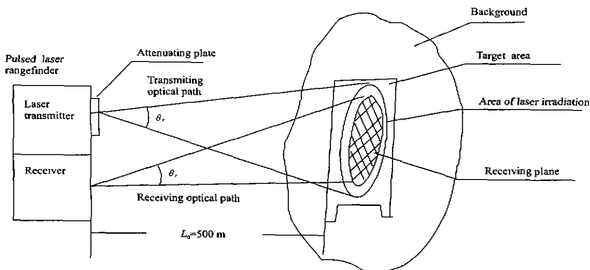
图 6 脉冲激光测距仪 P_{\min} 和 S 的测试系统
