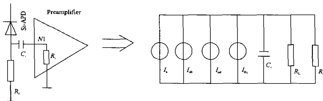
图 2 Si-APD 的工作原理及其等效电路图
