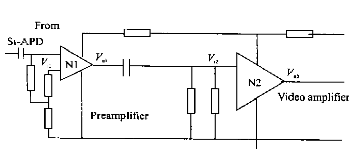
图 3 接收放大器等效电路
