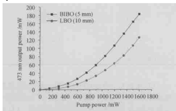
图 2 473 nm 蓝光输出随注入抽运功率的变化
