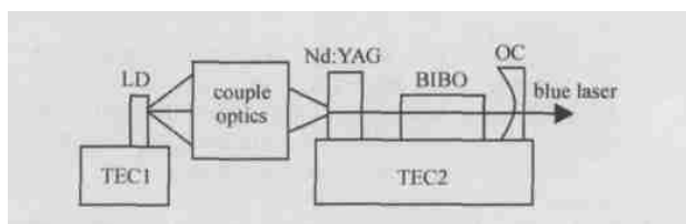
图 1 实验装置
