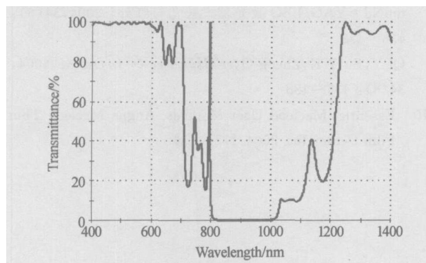
图4 平凹输出镜左端面膜系透射曲线
