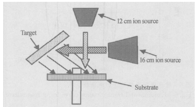
图5 双离子束溅射沉积薄膜系统
