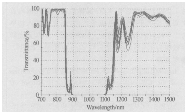
图3 相对标准差 1.5% 的误差分布曲线
