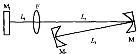
图 2 折叠腔设计示意图
