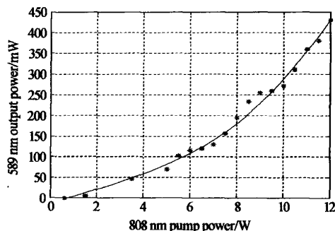
图 4 589 nm 和频光输出功率随入射抽运功率变换关系
