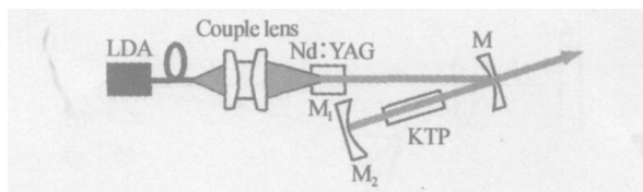
图 1 589 nm 激光器实验装置
