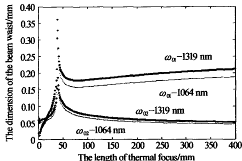
图 3 各分臂光腰随热焦距的变化
