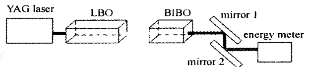
图3 产生三次谐波的实验装置
