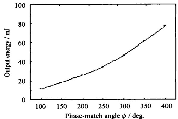
图4 BIBO 三次谐波 355 nm 输出能量随 1064 nm + 532 nm 输入能量的变化关系
