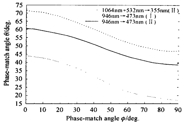
图2 BIBO 晶体 1064 nm 三次谐波相位匹配角和 946 nm 倍频相位匹配角
