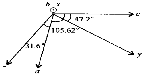
图1 BiB 3 O 6 晶体的光学主轴 ( x, y, z ) 与结晶学主轴 ( a, b, c ) 的相对取向
