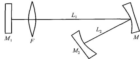
图 1 折叠腔示意图
