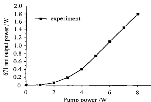
图3 671 nm 红光输出功率随抽运功率的变化
