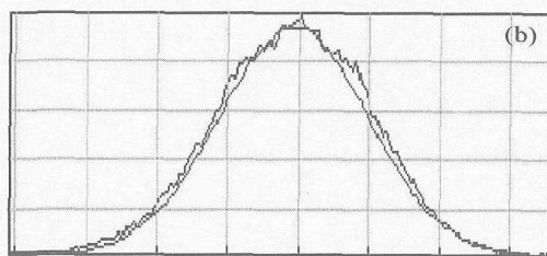
图 4 远场光斑照片(a)和能量近高斯函数分布曲线(b)
