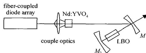
图 2 光纤耦合 LD 抽运 Nd:YAG/LBO 红光激光器示意图
