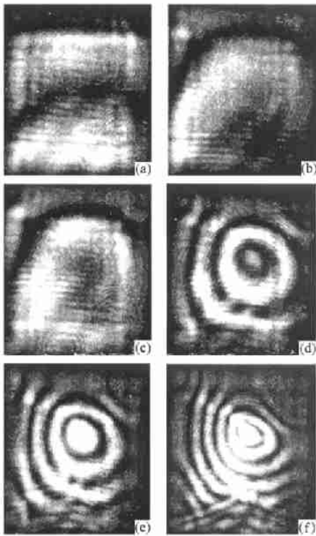
图 2 晶体前后表面之间的干涉图样 (a) —(f) 的抽运功率依次为 0, 2.4, 3.8, 7.0, 8.6 和 12.0W
