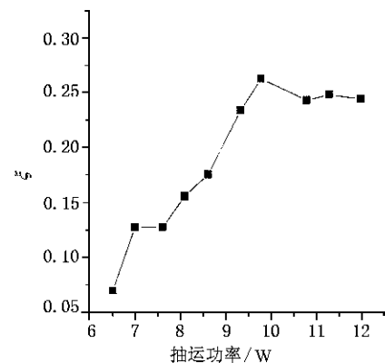
图 4 端面效应在整个热透镜效应中所占的比重随抽运功率的变化关系
