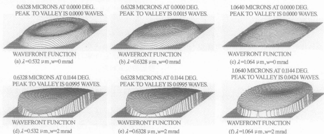
图 3 三种波长的波像差
