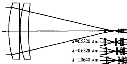
图2 光学系统 Fig.2 Optical system
