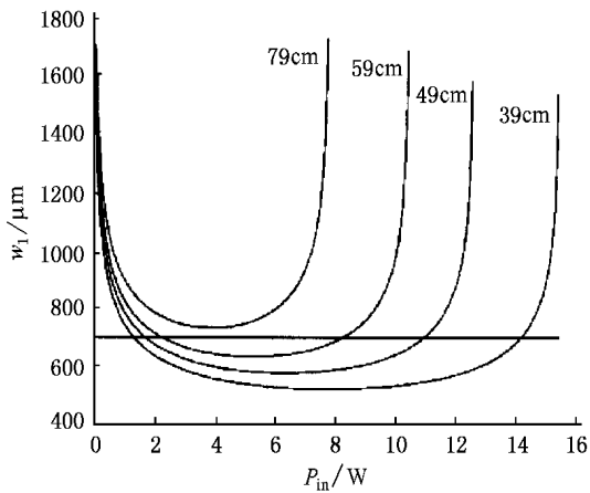
图3 振荡光基模光斑半径随抽运功率变化的关系曲线
