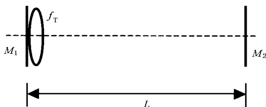
图 1 内含热透镜的平行平面腔
