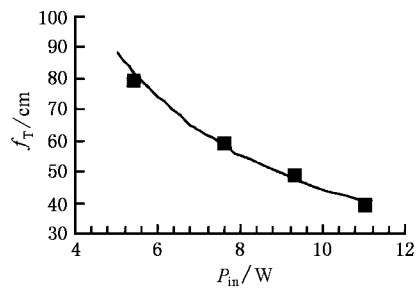
图6 不同抽运功率下的热透镜焦距
