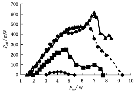
图5 不同腔长下输出功率随抽运功率变化曲线 为79cm, 为59cm, 为49cm, 为39cm
