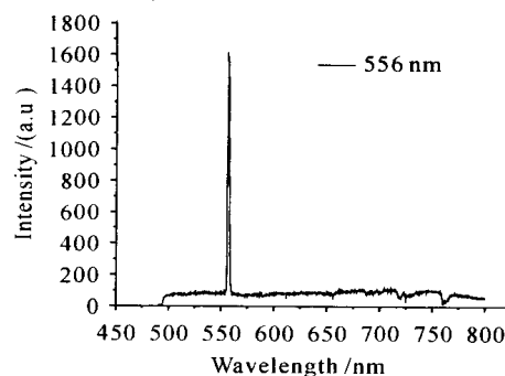
图 6 倍频光的输出光谱图
