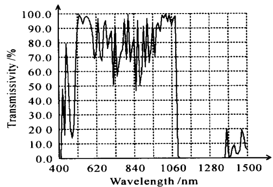
图 4 输出镜的透过率曲线
