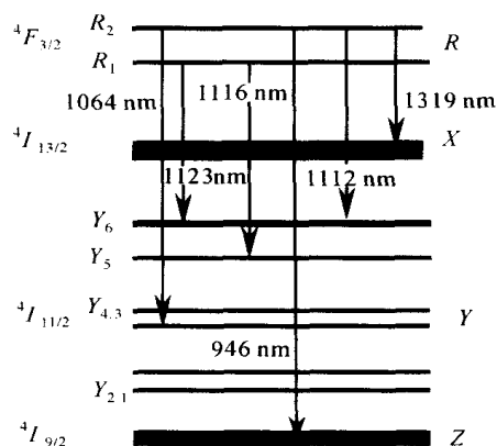
图 1 Nd:YAG 的能级图
