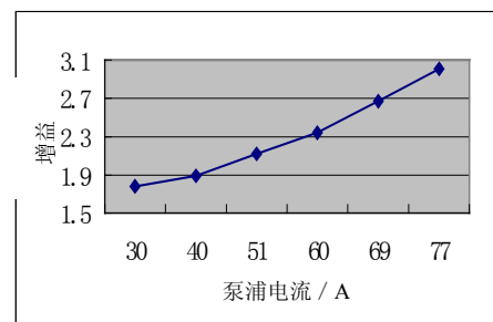
图 23 激光放大器的增益曲线
