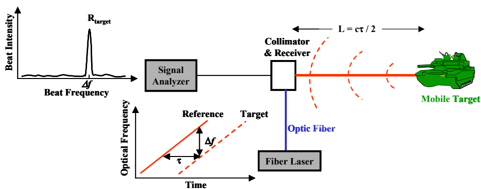
图 3：FMCW 技术在激光测距上的应用
