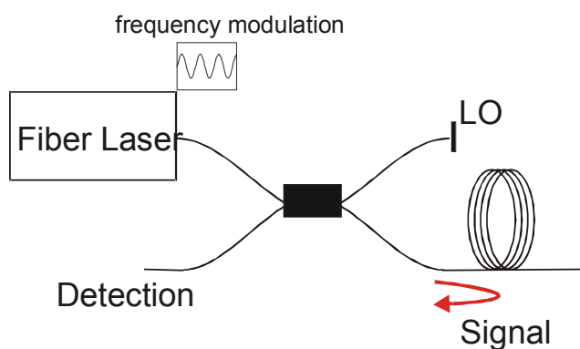
图 2：FMCW 技术原理图
