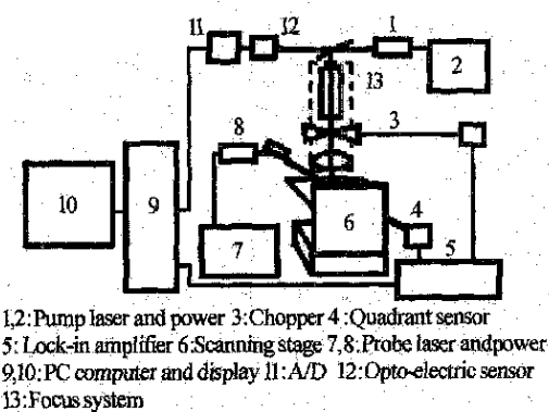
图 2 光热偏转实验检测装置
