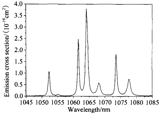
图 2 室温下 1.0at%Nd:YAG 陶瓷的发射截面 Fig. 2 Emission cross section spectrum of the 1.0at%Nd:YAG transparent ceramic
