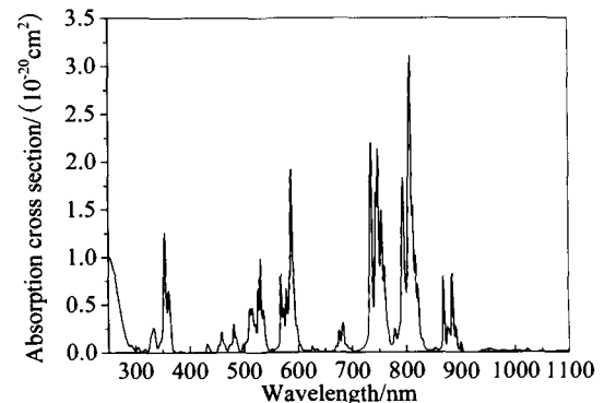
图 1 1.0at%Nd:YAG 透明陶瓷的吸收截面
