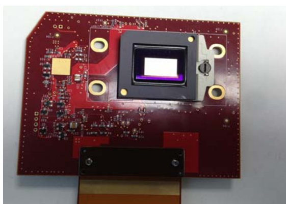
0.65" 1080p (1920x1080) DMD (S600 封装) 接口板
