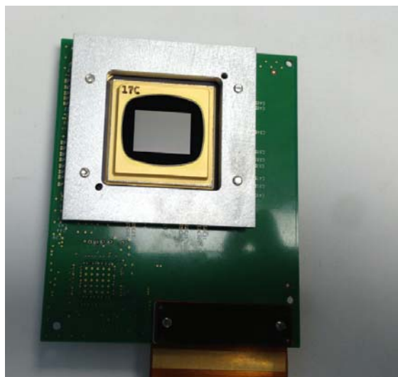
0.95" SXGA+(1400x1050) DMD 接口板
