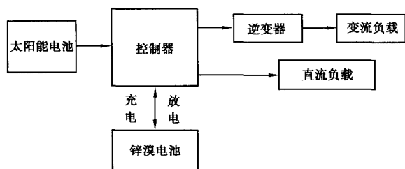
图 1 照明系统结构框
