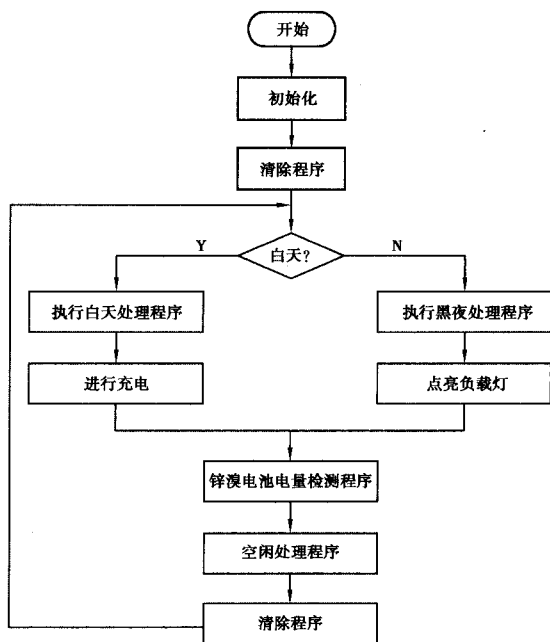
图 6 照明系统主程序流程
