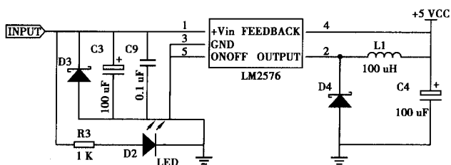
图 4 电源电路
