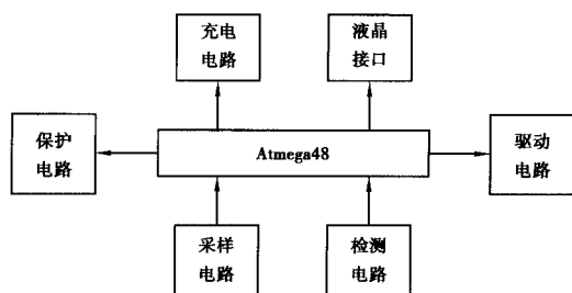
图 3 硬件系统结构框
