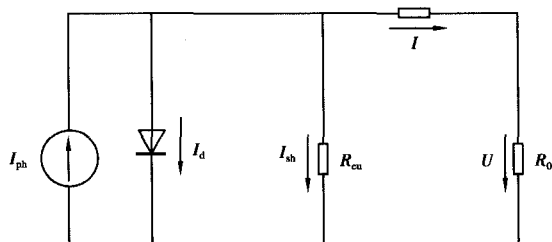
图 2 太阳能电池等效电路
