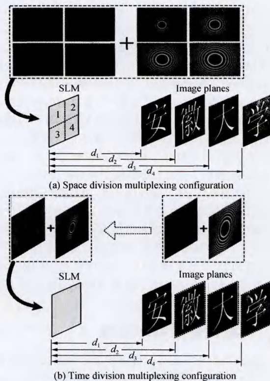
图 2 多平面全息投影示意图
