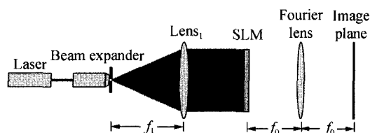
图 1 全息投影系统原理
