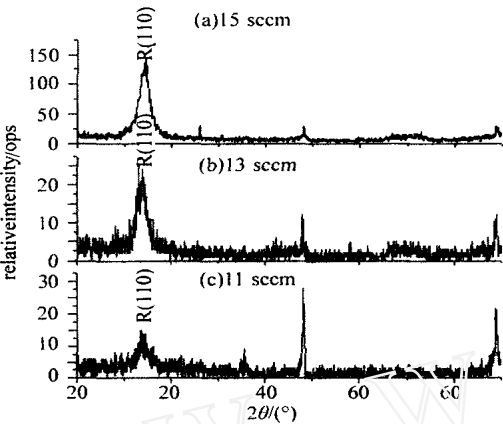
图 6 不同氧流量下制得的 TiO 2 薄膜 XRD 谱图 Fig. 6 XRD pattern of the TiO 2 thin films grown at different O 2 flow
