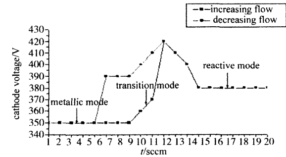
图 2 反应磁控溅射制备 TiO 2 薄膜的迟滞回线 Fig. 2 The hysteresis behaviour of DC reactive sputtering of TiO 2
