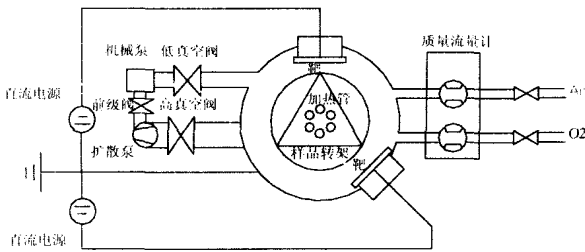
图 1 磁控溅射设备结构示意图 Fig. 1 Schematic diagram of the experimental apparatus
